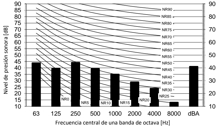
Modo refrigeración
