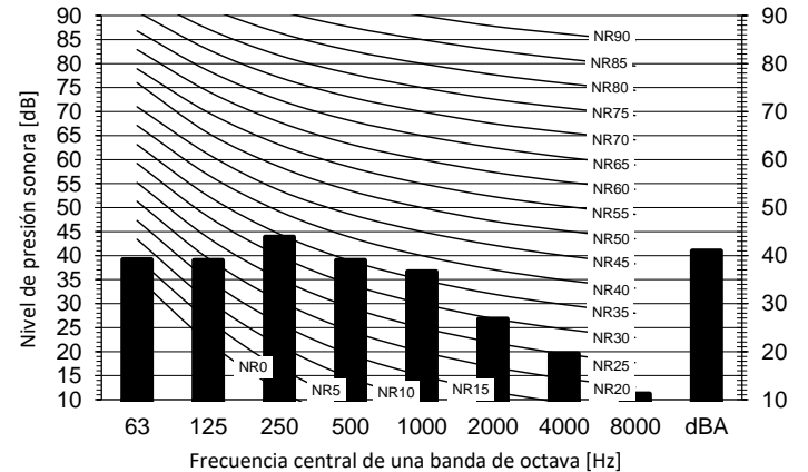
Modo calefacción
