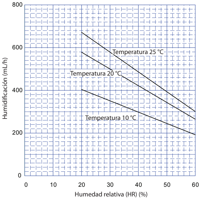
Humidificación frente a Humedad relativa
