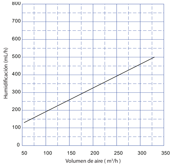
Humidificación frente a Volumen de aire
