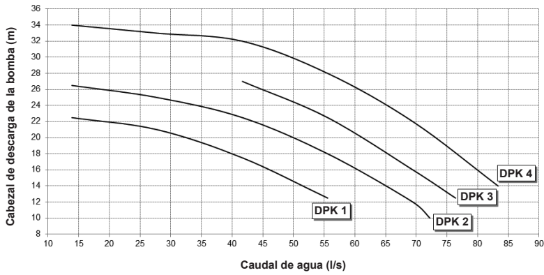
Bomba doble (2 polos) - Cabezal de descarga
