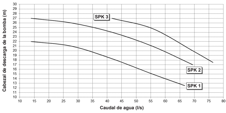
Bomba sencilla (2 polos) - Cabezal de descarga
