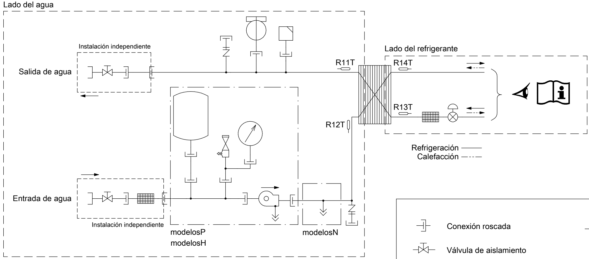
Enfriador tipo inverter pequeño - combinación de módulo exterior
