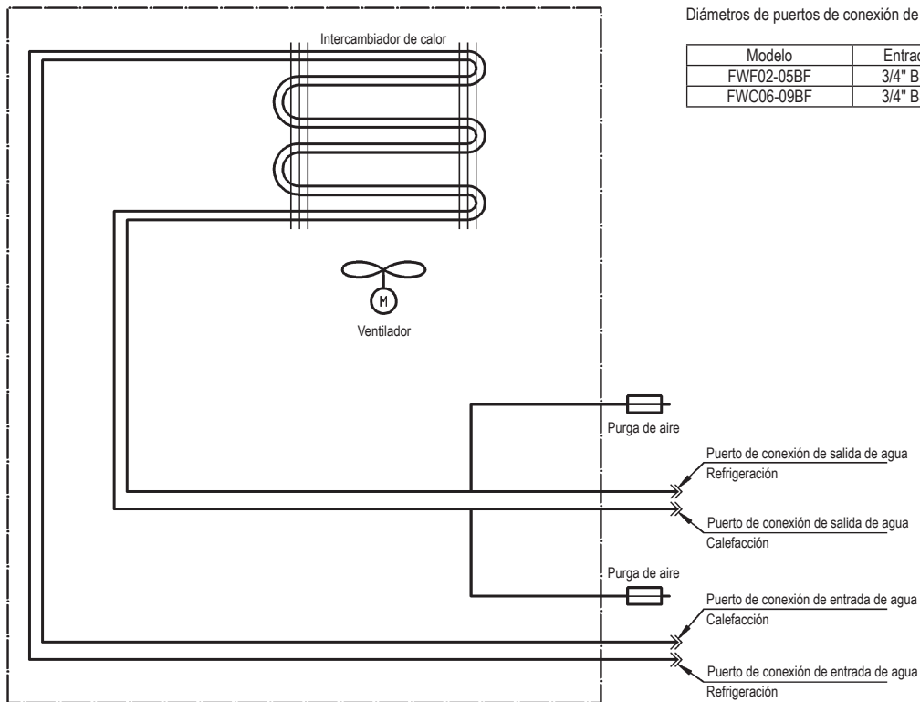
Diámetros de puertos de conexión de tubería de agua
