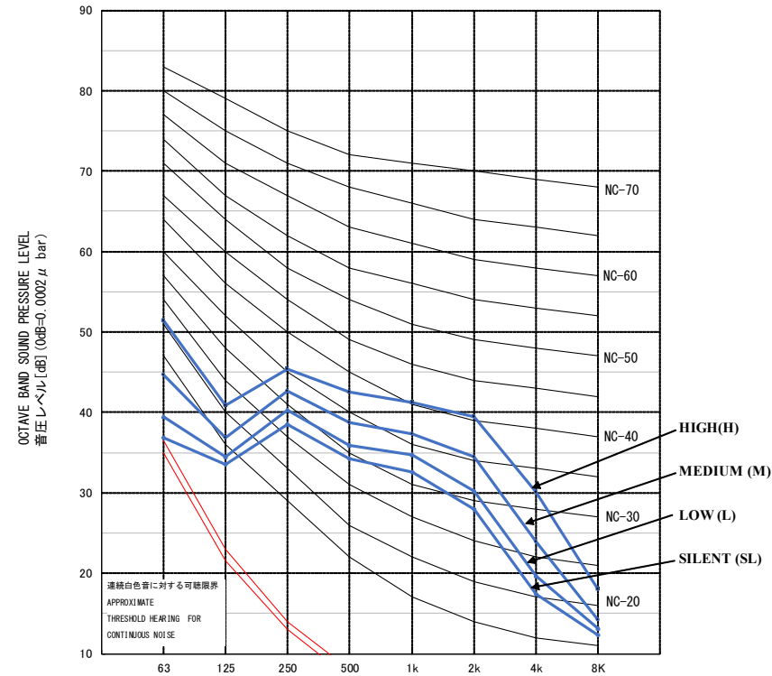
I E C オクターブバンド中心周波数 OCTAVE BAND CENTER FREQUENCY (Hz)
