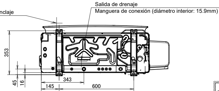
Vista inferior
