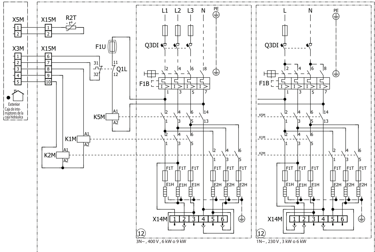
(1) Diagrama de conexiones
