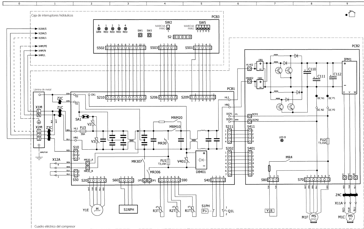
Cuadro eléctrico del compresor
