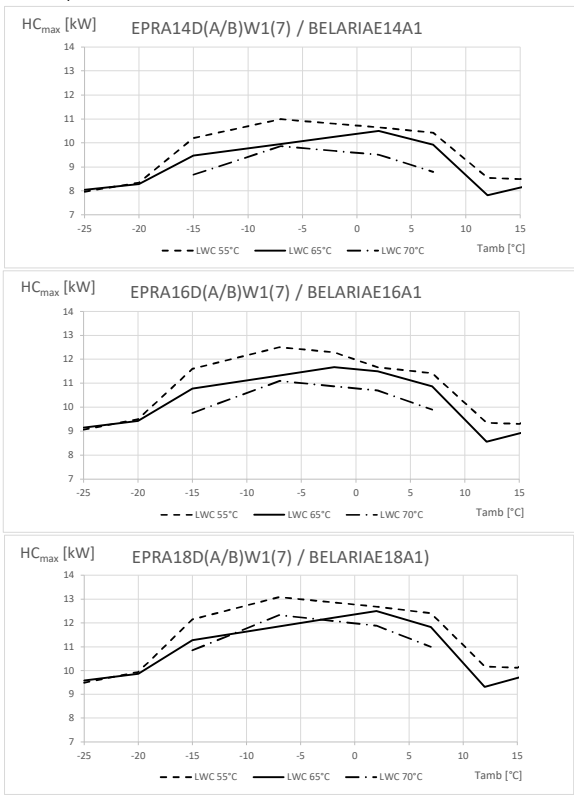
Capacidad de calefacción máxima - valores máximos
