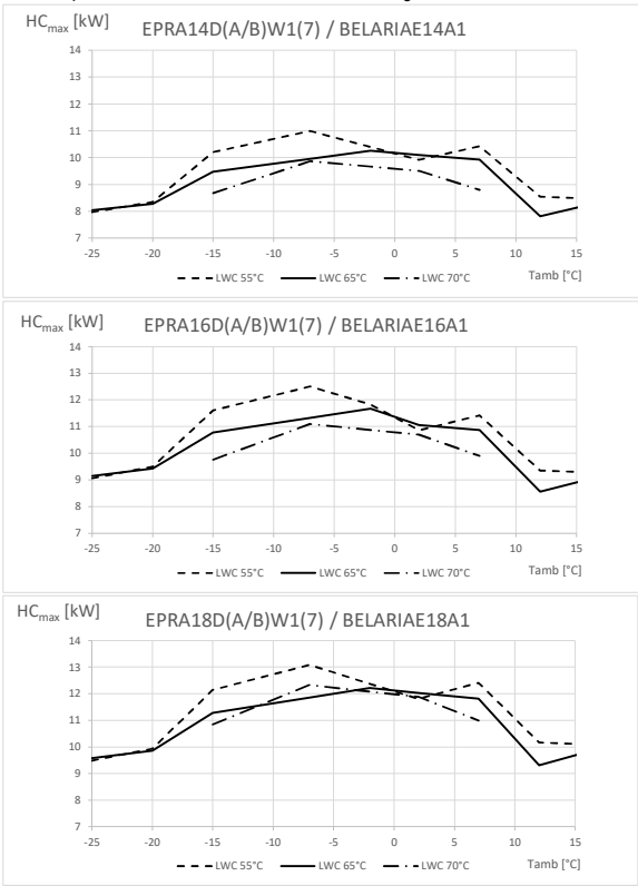
Capacidad de calefacción máxima - valor integrado
