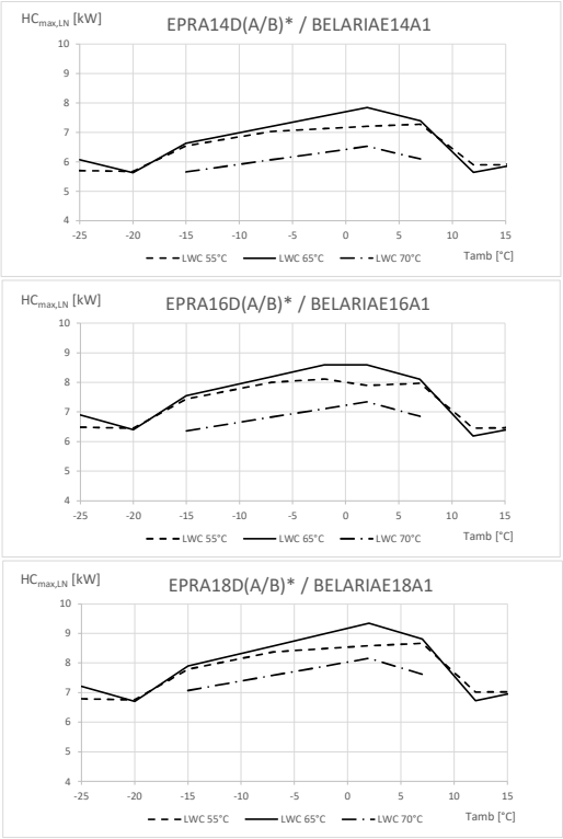
Capacidad de calefacción máxima - valores máximos
