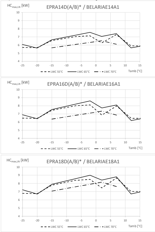
Capacidad de calefacción máxima - valor integrado
