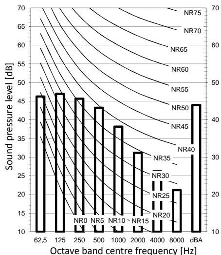
ERGA06*
