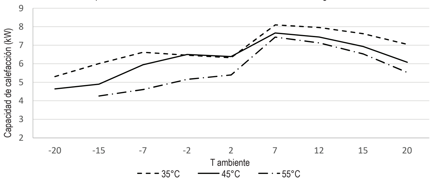
Capacidad de calefacción máxima ERGA08EAV3: Valores integrados
