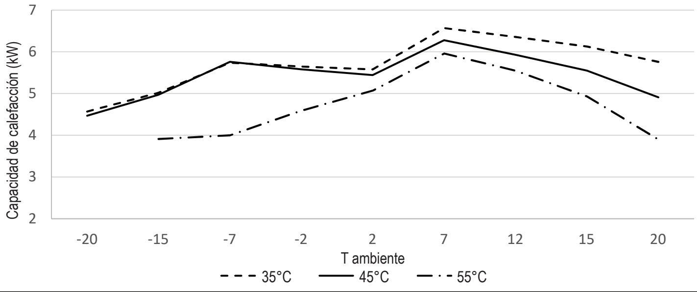
Capacidad de calefacción máxima ERGA06EAV3: Valores integrados
