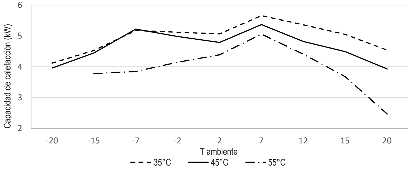
Capacidad de calefacción máxima ERGA04EAV3: Valores integrados
