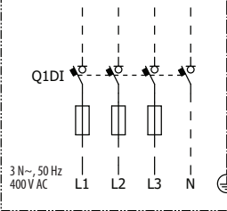
voor *6WN (3 N~, 400 V, 6 kW) en *9WN (3 N~, 400 V, 9 kW)
