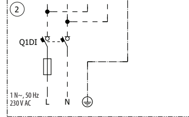
voor *6V3 (1 N~, 230 V, 6 kW)
