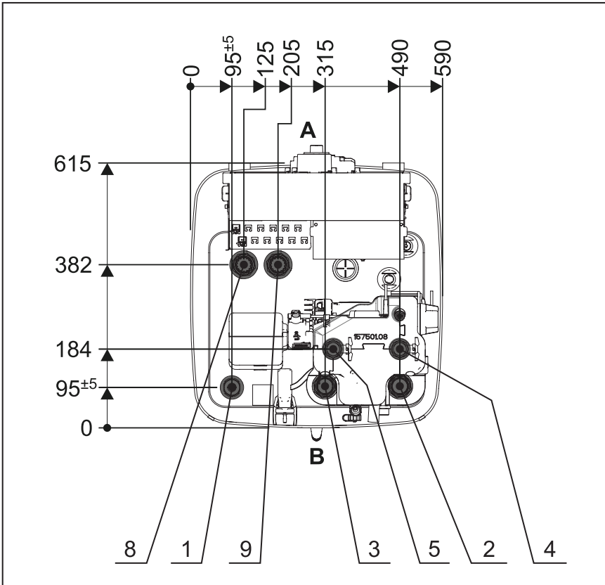
Dimensiones, parte superior de la unidad - ETS(X/H)B16P30D
