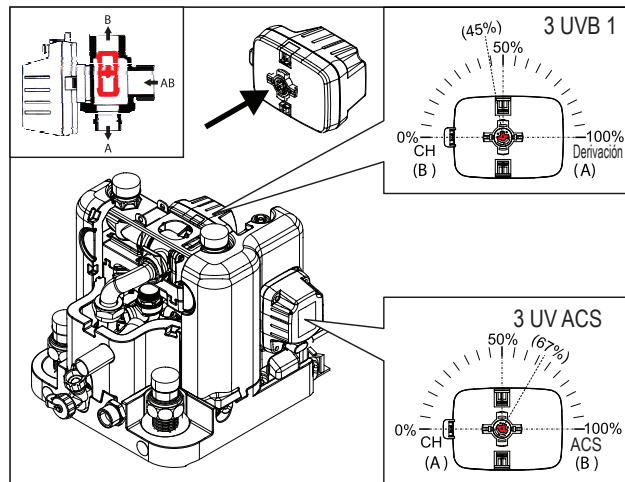
Válvula de desviación de 3 vías de función
