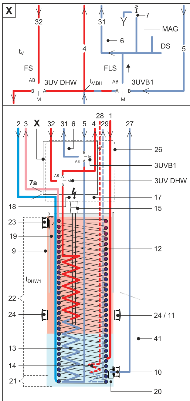
Configuración y componentes – configuración interior ETS(X/H)
