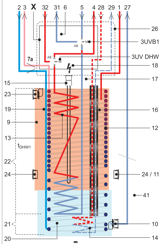
Configuración y componentes - configuración interior ETS(X/H)(B)16P50D (1)
