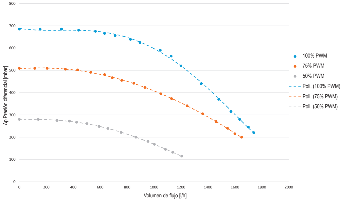
Curva ESP, modelos bivalente de 500 litros
