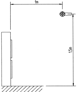
Lugar de la medición (Lado de descarga)
