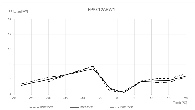
Capacidad de calefacción máxima - valor integrado
