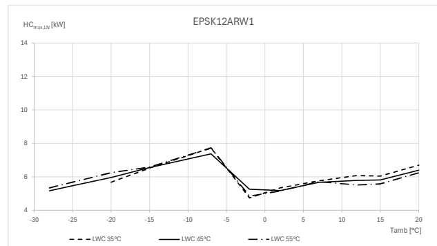
Capacidad de calefacción máxima - valores máximos
