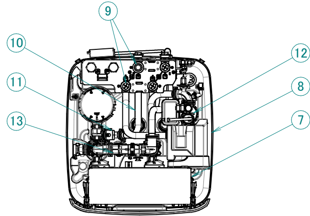
Vista superior Sin cubierta
