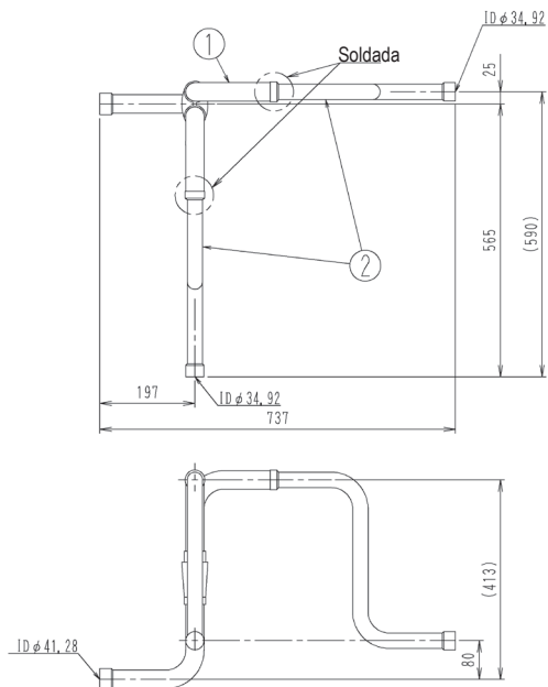
Conexión delantera
