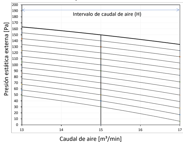
Características del ventilador (2)
