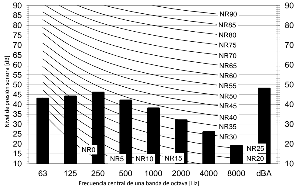
Modo refrigeración
