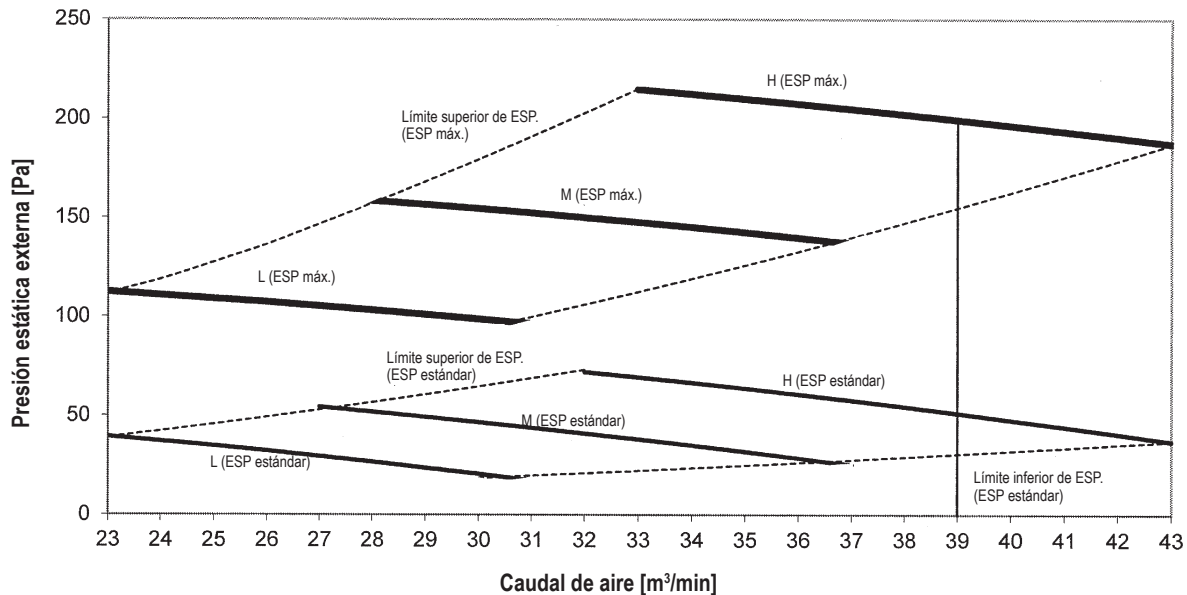
Características del ventilador (1) (1)
