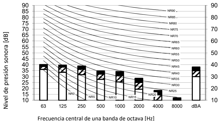
Modo refrigeración
