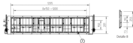
Vista A-A
