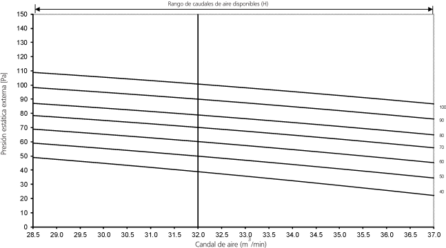
Características del ventilador (2) (Ajuste en la obra con el mando a distancia)
