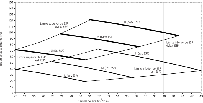
Características del ventilador (2) (Ajuste en la obra con el mando a distancia)
