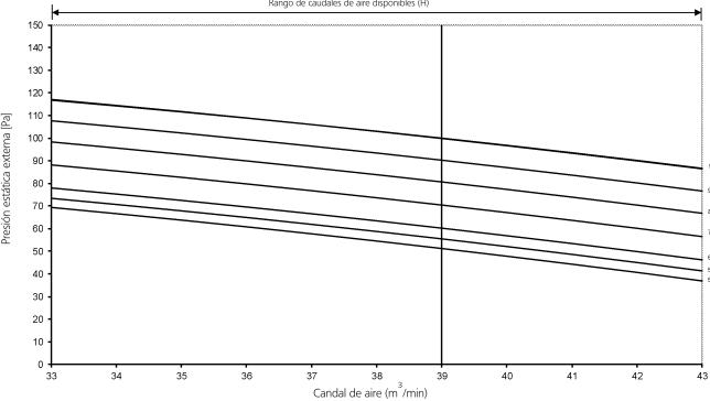
Características del ventilador (2) (Ajuste en la obra con el mando a distancia)
