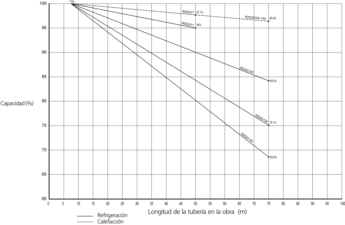
Capacidad en función de la longitud de tubería en la obra para el inverter
