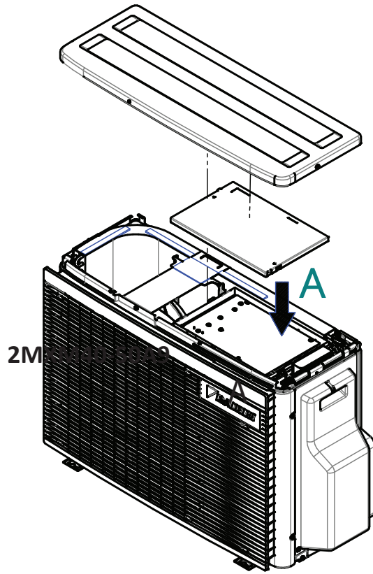
Desmontaje de la unidad
