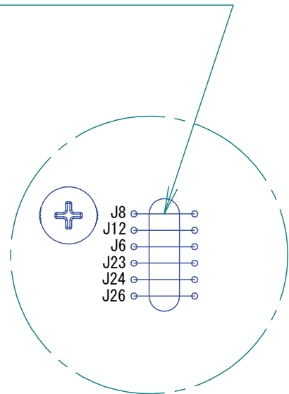
Detalle B
