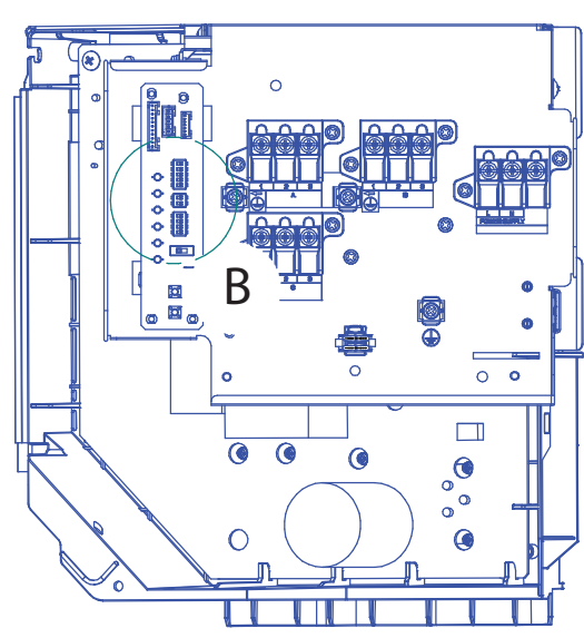
Vista de flecha A Conjunto de comp. elect.
