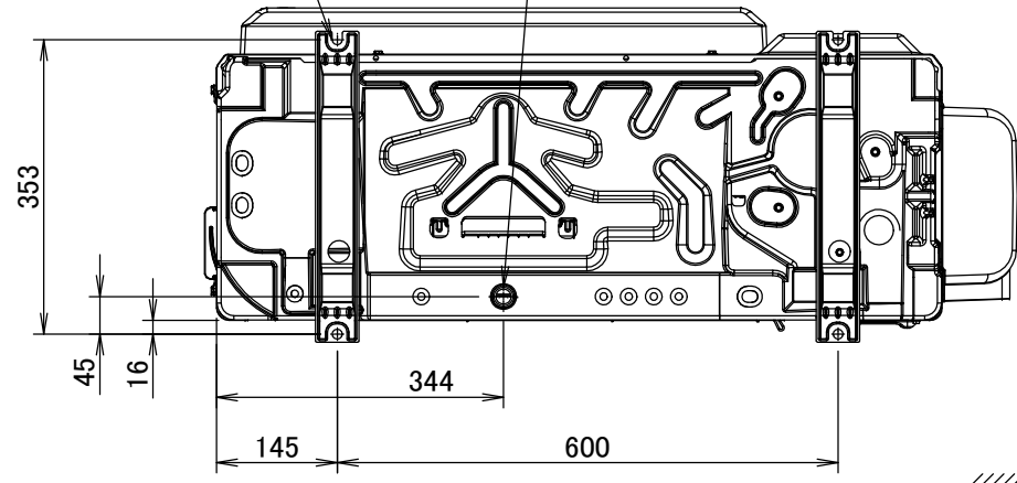
Vista inferior
