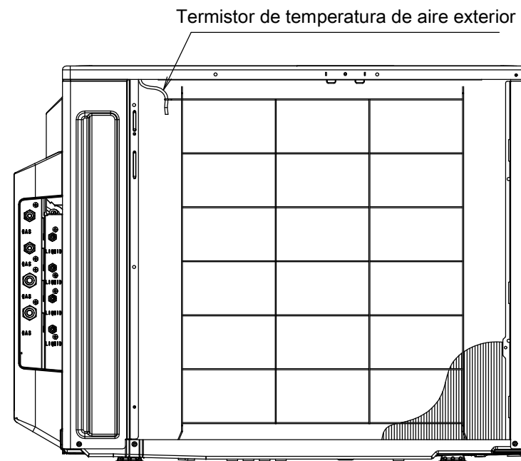
Vista trasera
