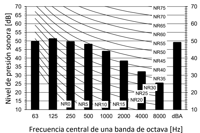
Modo calefacción
