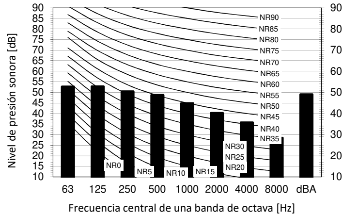
Modo calefacción
