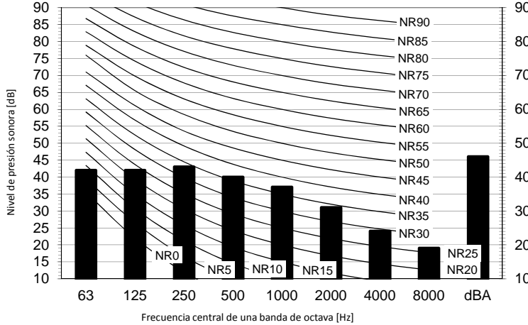
Modo refrigeración
