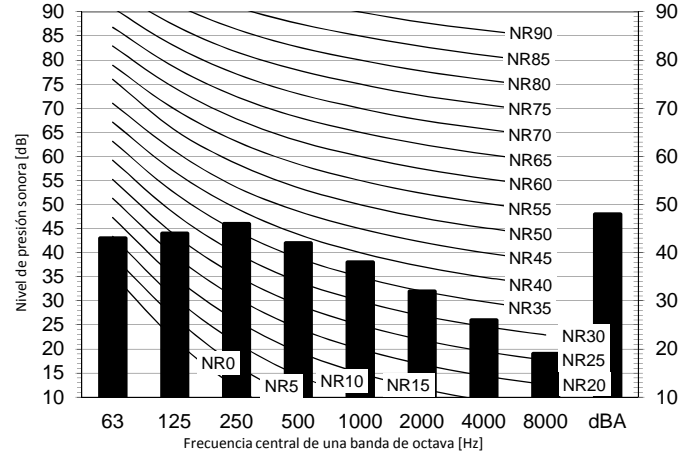
Modo calefacción
