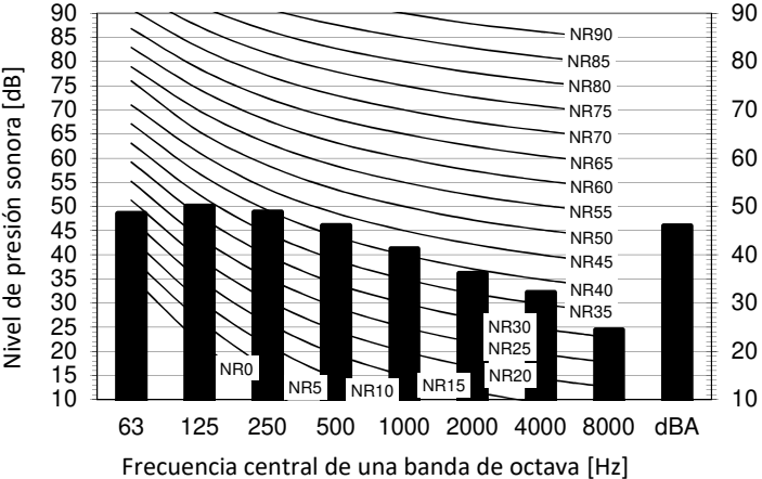
Modo refrigeración
