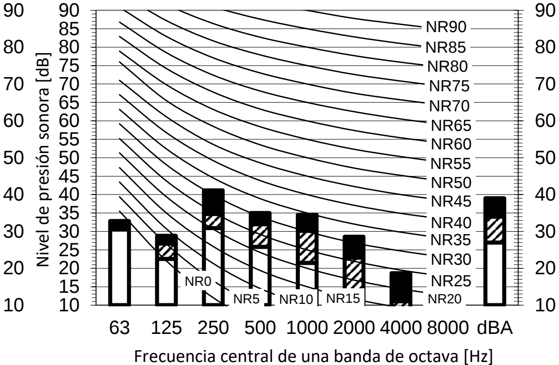
Modo calefacción
