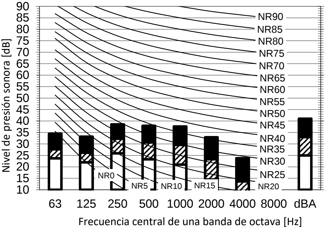
Modo refrigeración
