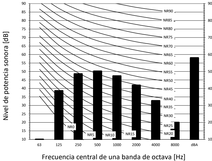
Modo calefacción
