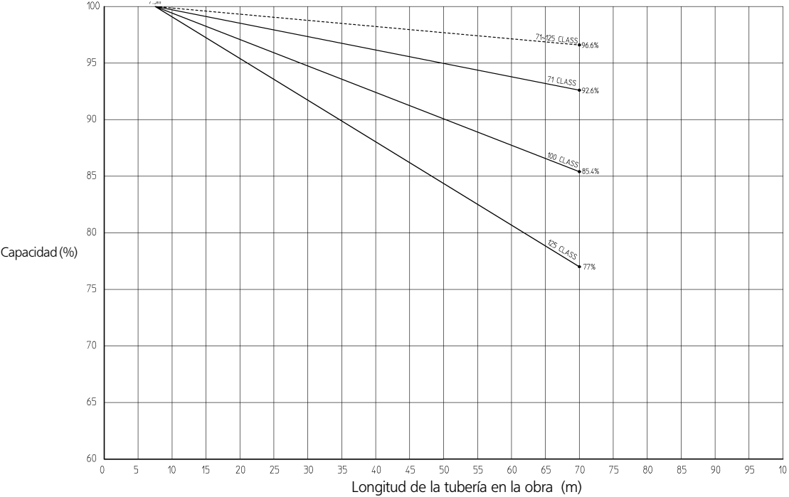
Capacidad en función de la longitud de la tubería en la obra sin inverter
