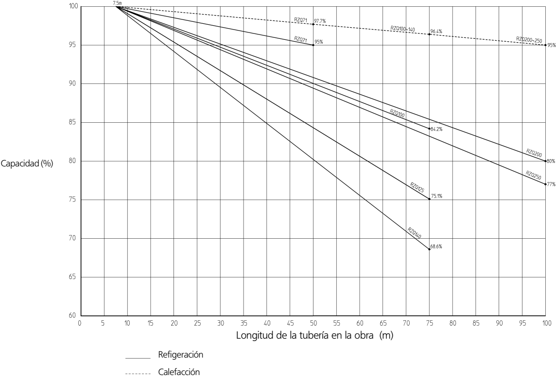
Capacidad en función de la longitud de la tubería en la obra sin inverter
