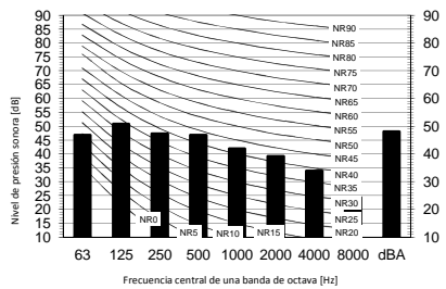
Modo calefacción
