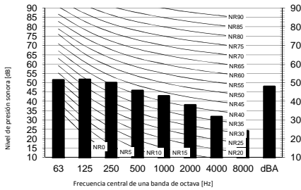
Modo refrigeración
