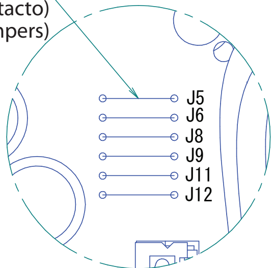
Detalle B
