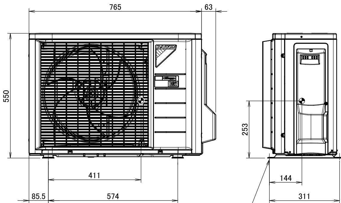
Orificio de pernos para base
