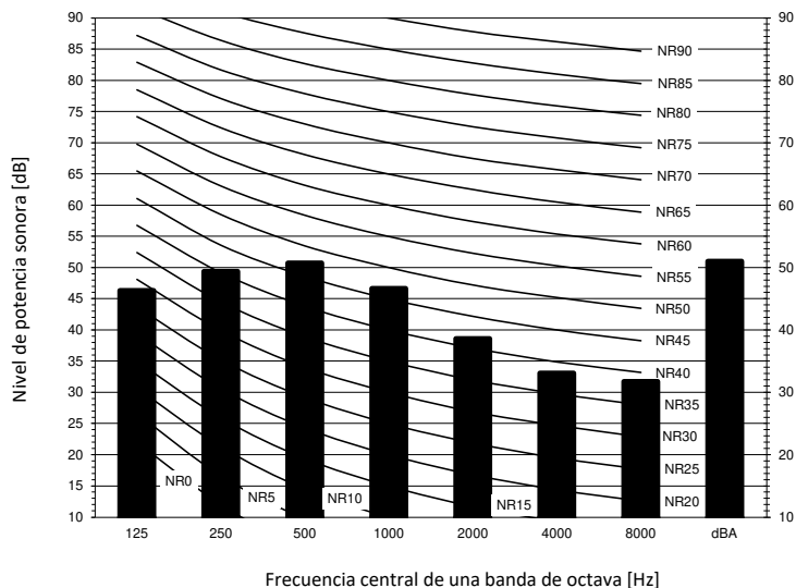
Modo refrigeración
