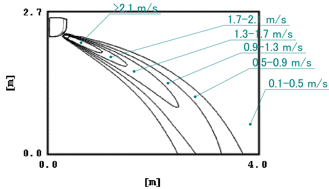
Distribución de velocidad del aire (calefacción) Sentido de circulación del aire: vertical
