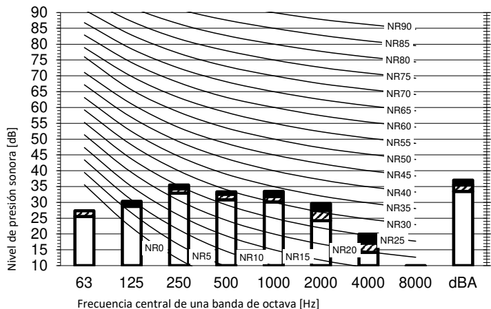
Modo refrigeración
