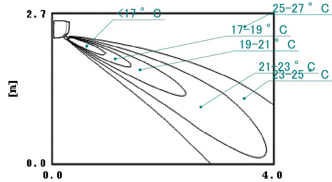
Distribución de temperatura del aire (refrigeración) Sentido de circulación del aire: horizontal
