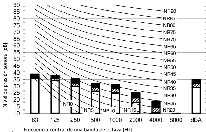
Modo refrigeración
