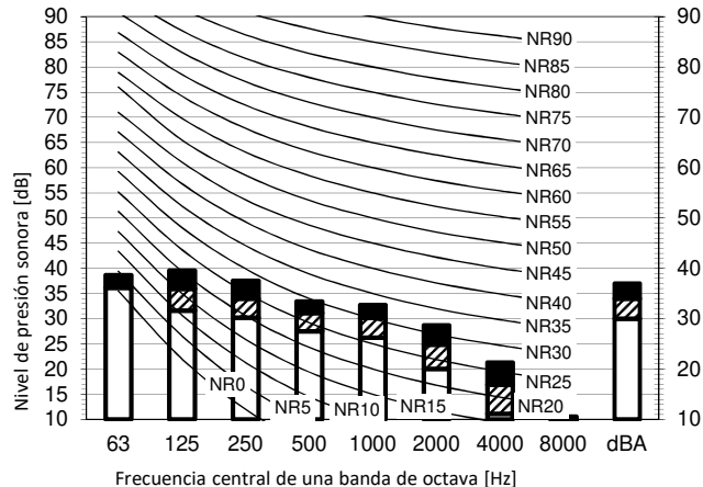
Modo calefacción
